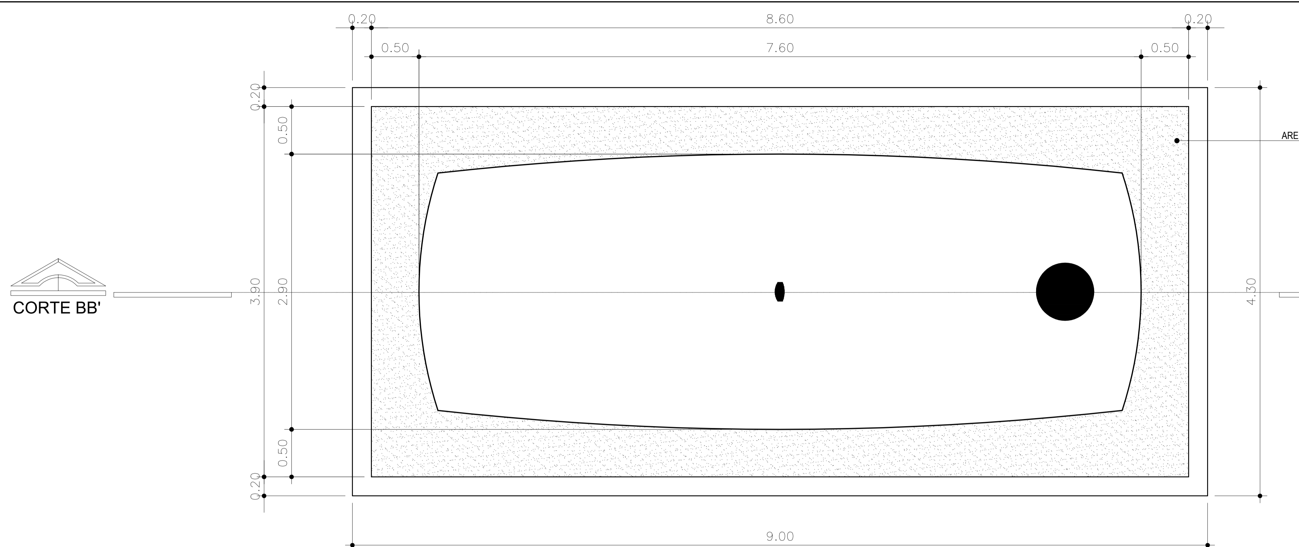
PLANTA BAIXA DA CAVIDADE PARA CISTERNA
